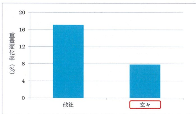
グラフ1 水浸漬後の重量変化率
